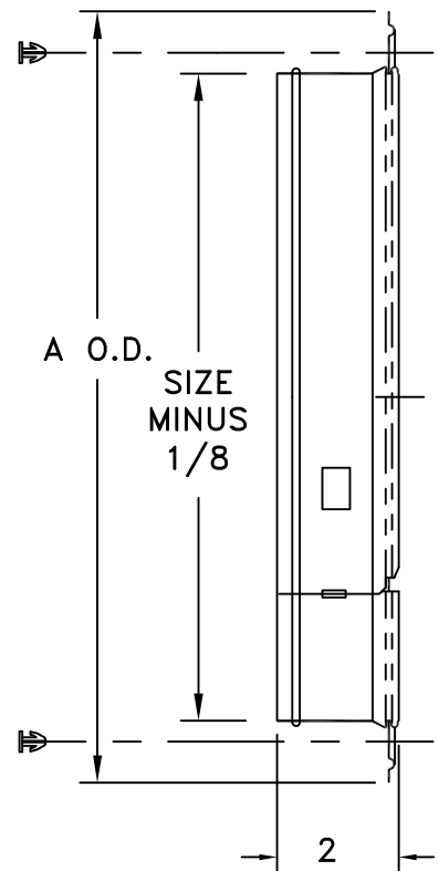
SECTION A-A
